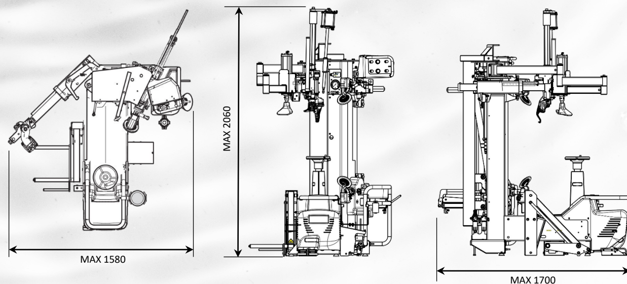
寸法図
